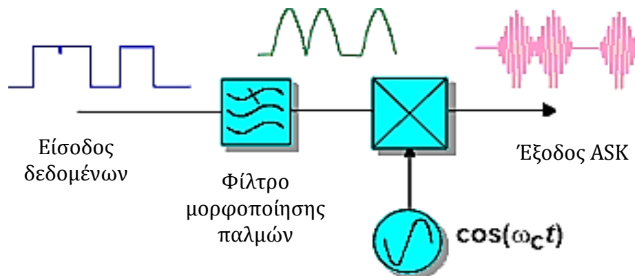
Διαμορφωτής BASK
