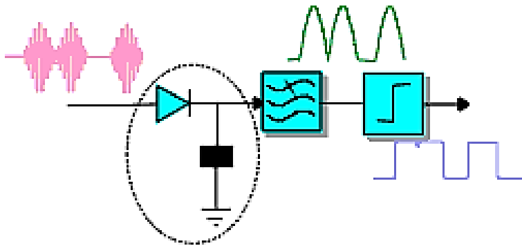
Ασύμφωνος αποδιαμορφωτής BASK
